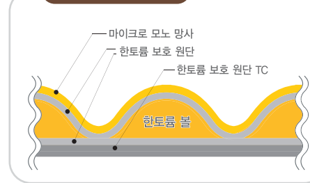
한토름 상판 단면도
